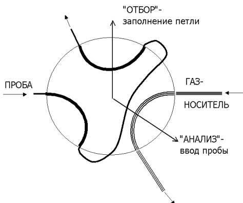
Рис. 8. Схема поворотного крана-дозатора с дозирующим объемом в виде трубки, установленной на вращающейся втулке
