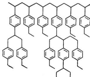
Рис. 6. Структурная формула порапака
