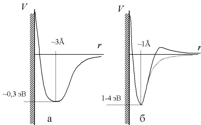
Рис. 2. Потенциальная энергия взаимодействия молекул с поверхностью в случаях: а) - физической адсорбции, б) - химической адсорбции
