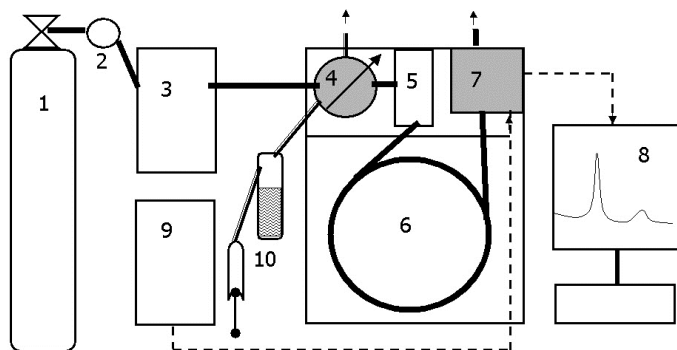
Рис. 7. Блок-схема хроматографа: 1—баллон с газом-носителем, 2—редуктор, 3—блок подготовки газов (БПГ), 4—кран-дозатор, 5—испаритель, 6—колонка в термостате, 7—детектор, 8—управляющий компьютер, 9—блок питания детектора (БПД), 10—система парового ввода пробы (шприц, сосуд с парами)
