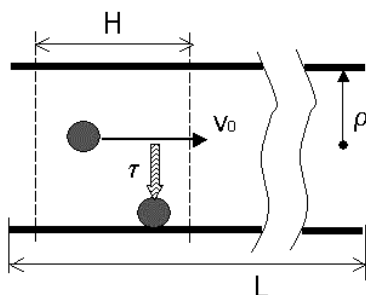
Рис. 3. Иллюстрация понятия высоты эквивалентной теоретической тарелки (ВЭТТ)
