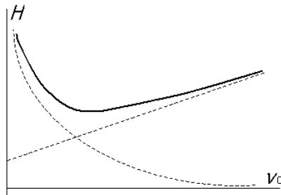
Рис. 4. Зависимость ВЭТТ от скорости потока газа-носителя, описываемая уравнением Ван-Деемтера (42)
