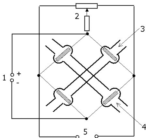
Рис. 9. Пневмоэлектрическая схема ДТП: 1—питание моста от БПД, 2—установка нуля, 3—чистый газ-носитель (сравнительный поток), 4—ПФ из колонки (измерительный поток), 5—сигнал детектора
